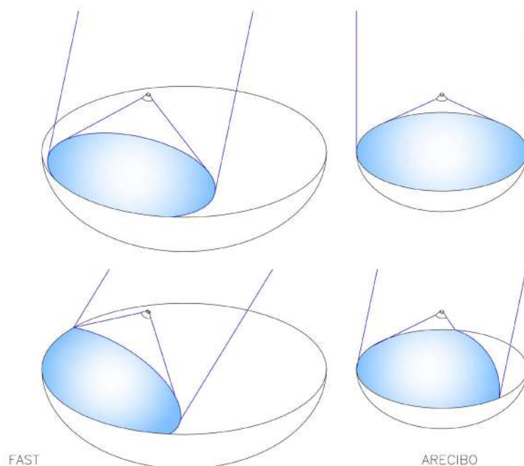
Figura 149 - Desenho comparativo entre o FAST e o radiotelescópio de Arecibo. A antena do FAST é muito maior, mas o observatório coleta a radiação de apenas uma parte da antena (em azul), muito similar à capacidade de Arecibo. O telescópio pode, no entanto, observar uma área muito mais ampla do céu do que a antena de Porto Rico, como ilustra a parte inferior da figura. Desenho: Francisco Conte.
