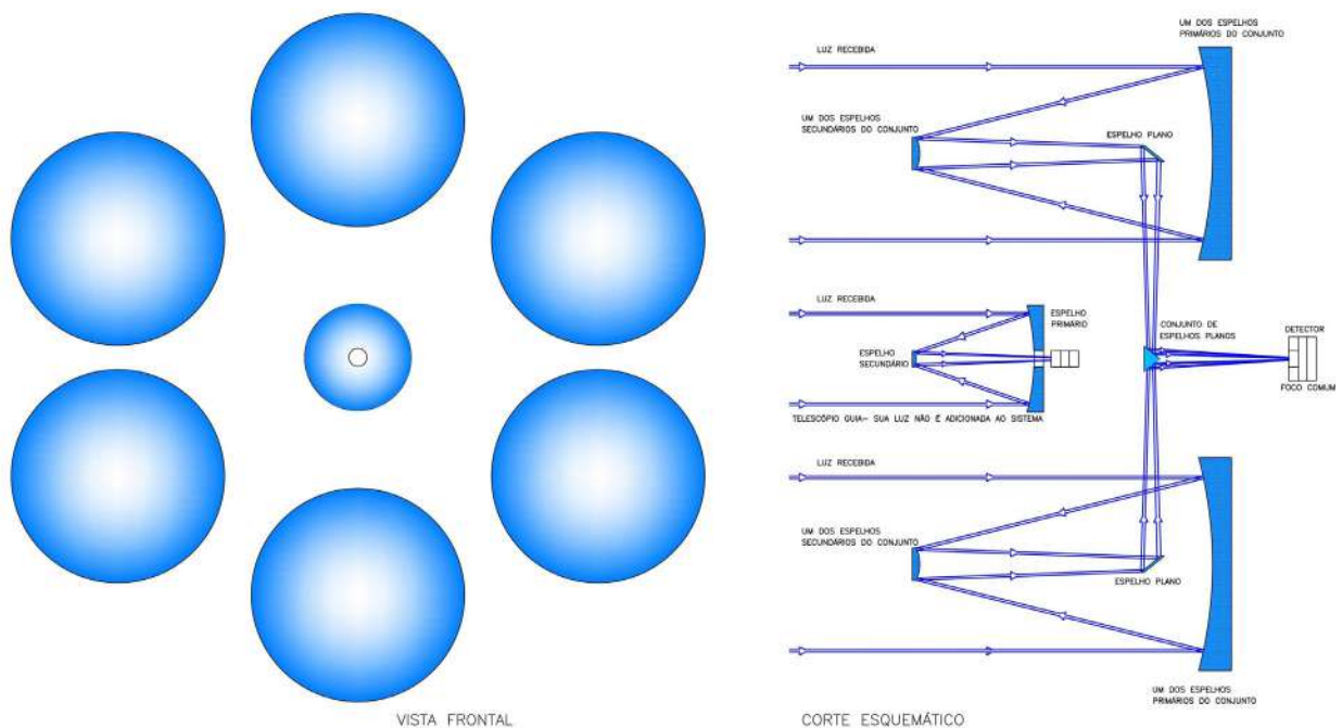
Figura 91 - Esquema óptico do MMT (Multiple Mirror Telescope), frontal e corte. O MMT foi um dos mais revolucionários telescópios da história, utilizando seis espelhos de 1,80 m, que equivaliam em área a um espelho de 4,50 m, por uma fração do custo. Foi também um dos primeiros telescópios a utilizar uma montagem altazimutal. Desenho: Francisco Conte.
