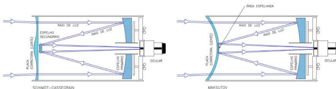
Figura 173 - Esquemas ópticos de dois telescópios catadióptricos: à esquerda um Schmidt-Cassegrain e à direita um Maksutov. Desenho: Francisco Conte.
