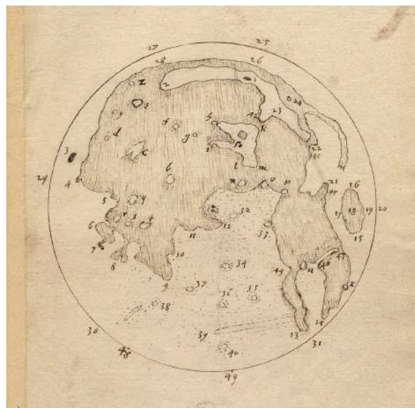
Figuras 7 e 8 - Desenhos da Lua feitos por Galileu (no alto) e Thomas Harriot. Como se pode observar, o desenho de Harriot é mais fiel ao relevo geral da Lua, mas os de Galileu, apesar de mais esquemáticos, apresentam detalhes mais definidos. Fonte: Wikimedia Commons.
