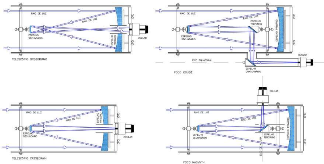
Figura 172 - Desenho de quatro esquemas ópticos de telescópios refletores: acima, à esquerda, um telescópio gregoriano; abaixo, à esquerda, um telescópio Cassegrain; acima, à direita, um telescópio com foco Coudé e abaixo, à direita, um telescópio com foco Nasmyth. Desenho: Francisco Conte.
