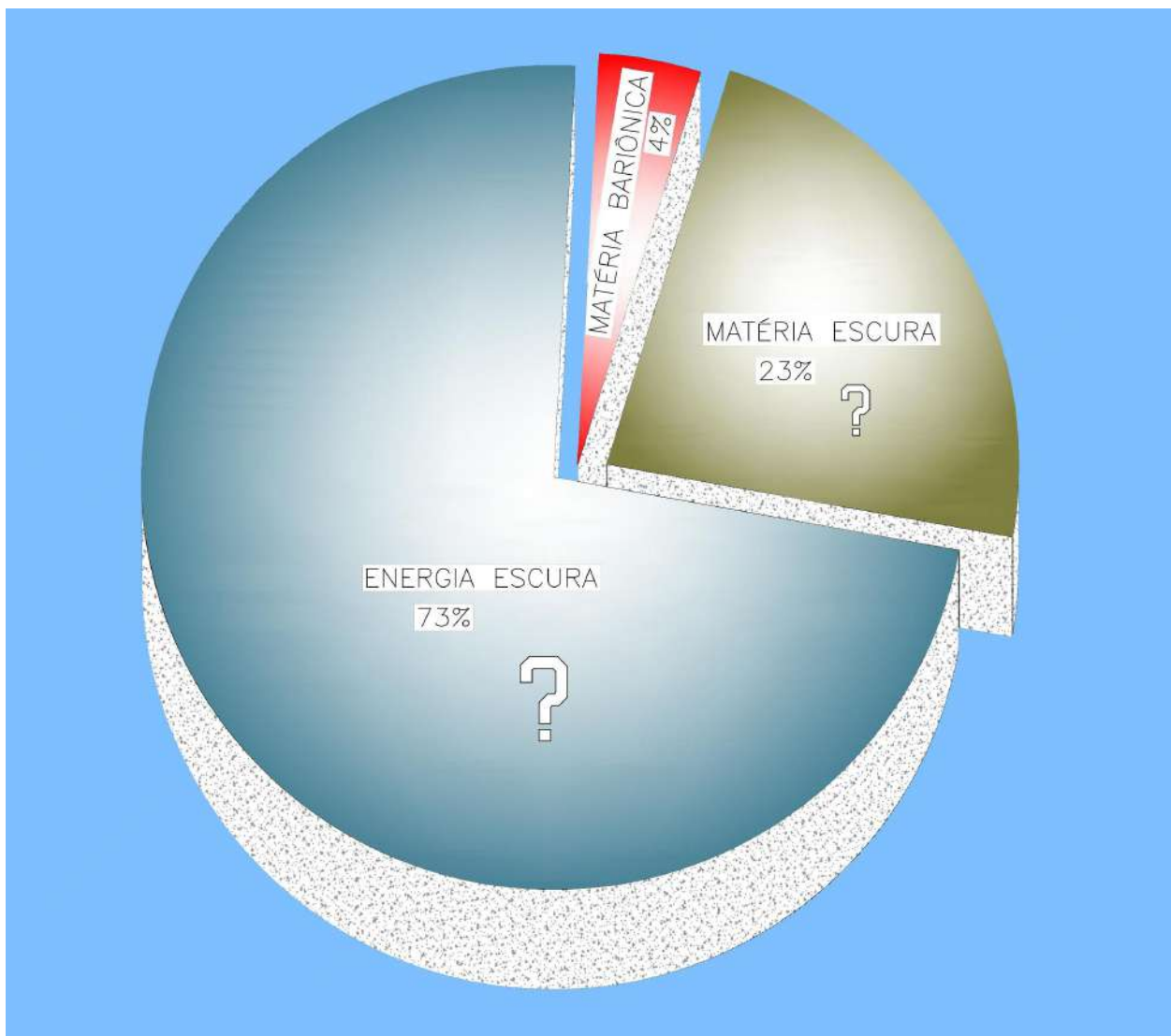
Figura 108 - Do que é feito o universo? Toda a matéria que podemos observar – galáxias, poeira, estrelas, neutrinos etc. – corresponde a apenas 4% do total de matéria e energia que compõem o nosso universo. Os restantes 96% do total são constituídos de matéria escura e energia escura, que ainda não sabemos exatamente o que são. Desenho: Francisco Conte.
