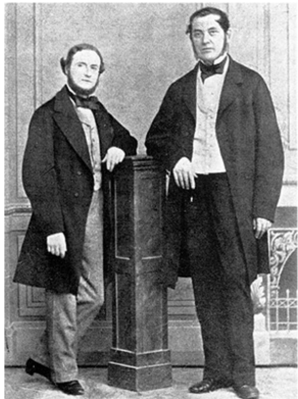
Figura 38 - Gustav Robert Kirchhoff e Robert Wilhelm Eberhard Bunsen, os pais da espectroscopia. Fonte: Wikimedia Commons.
