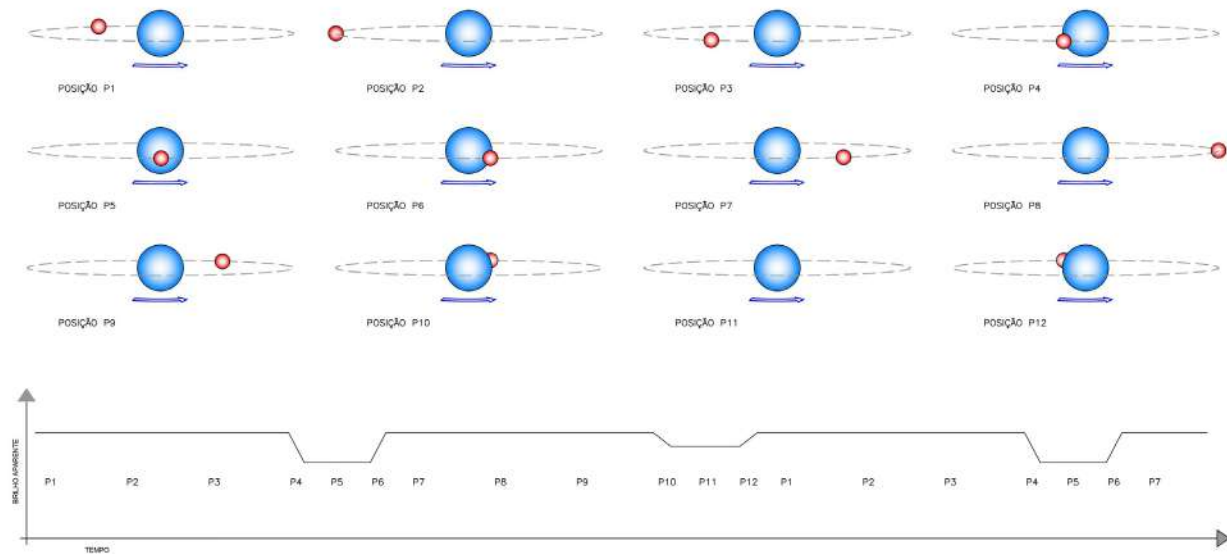
Figura 15 - Binárias eclipsantes: um sistema binário de estrelas, em que, eventualmente, uma passa pela frente da outra, com consequente redução do brilho total para o observador. Essa redução de brilho é diferente quando a estrela menos brilhante passa na frente ou atrás da estrela principal. Os dois eventos se repetem periodicamente, podendo ser prevista a data de um novo eclipse. Esse tipo de gráfico, que observamos na parte inferior da figura, onde foi plotado o brilho do objeto em função do tempo, é chamado de curva de luz. Desenho: Francisco Conte.
